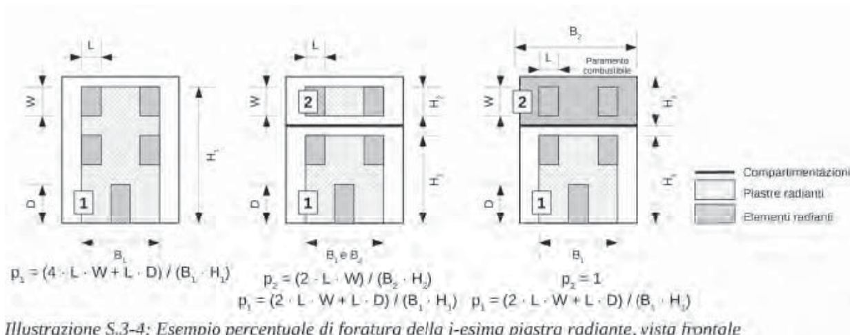
Illustrazione S.3-4: Esempio percentuale di foratura della i-esima piastra radiante, vista frontale
